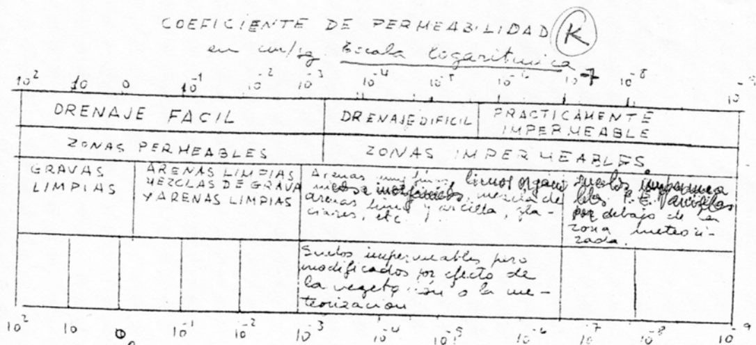
Fig 3-7 - 10 0 Clasificación de los suelos por su coeficiente de permeabilidad (según Casagrande y Fadum)
